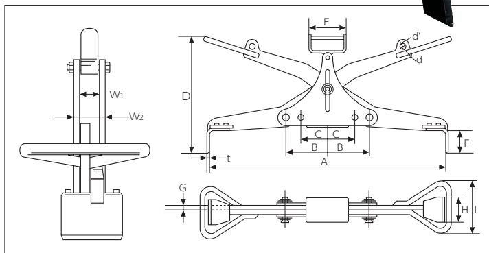
■ Table of Dimensions (Model : UGHC)
