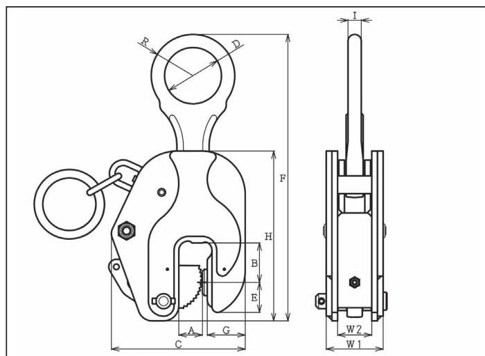
■ Table of Dimensions (Model : SL)
