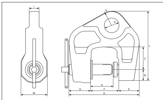
■Table of Dimensions (Model : SBC)
