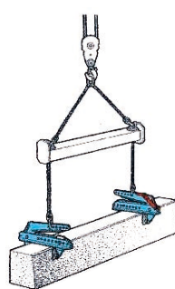
▲ Curbstones
