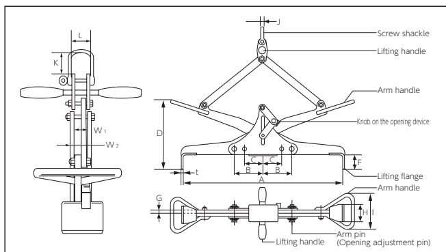
■ Table of Dimensions (Model : UGM)
